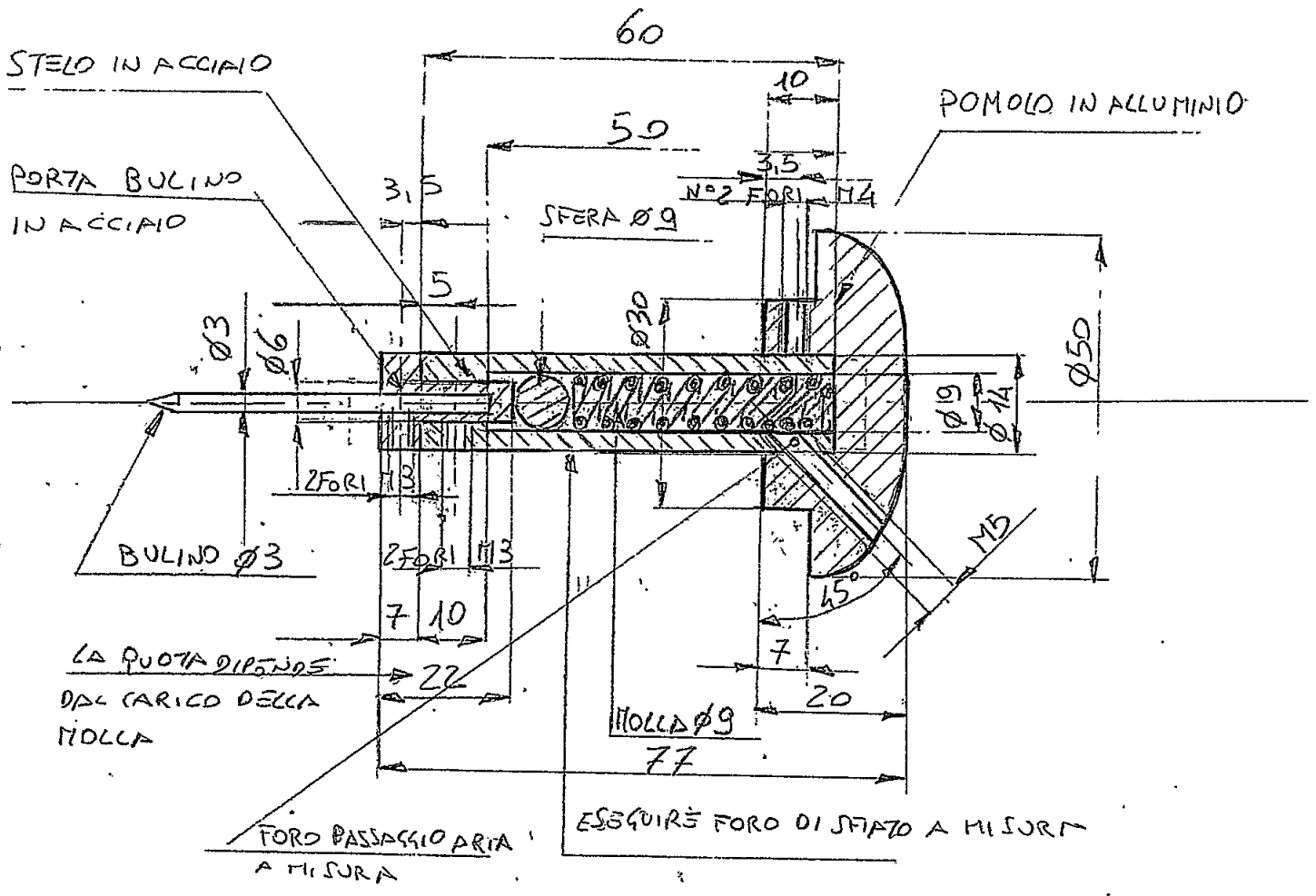
SCALA 1:1 ASSIEME BULINO PNEUMATICO VERSIONE PER BULINI STANDARD
